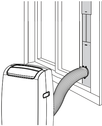
[좌우 여닫이 창(수평창) 설치 형태]
